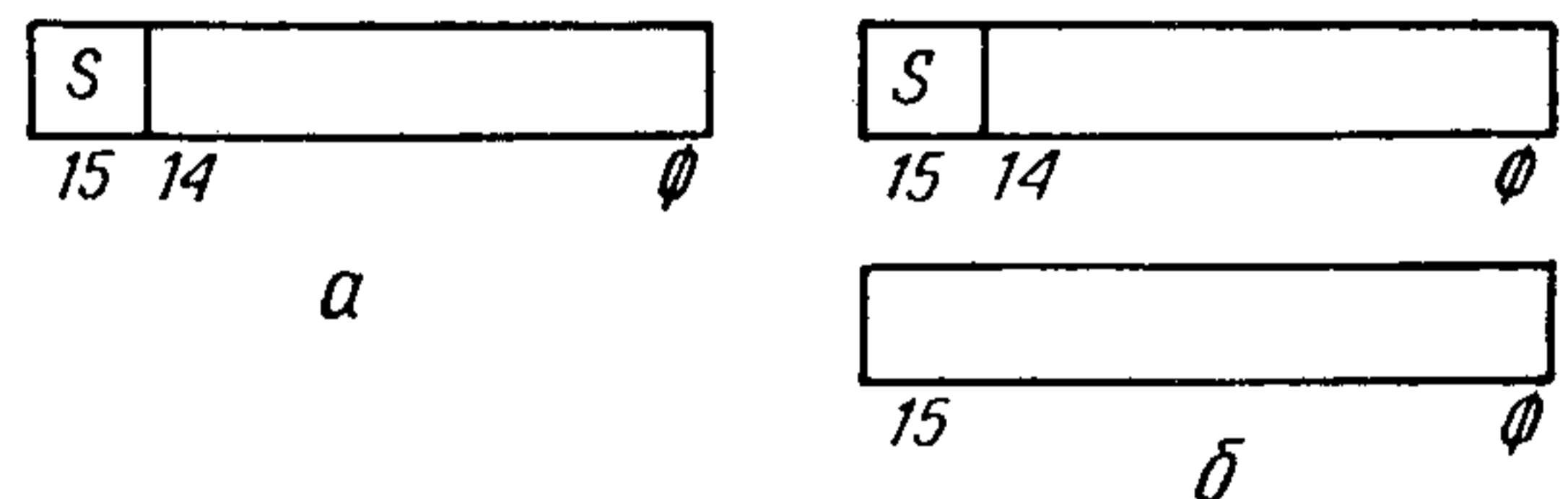
Рис. 36. Формат чисел с ФЗ, используемых в командах с ПЗ:
