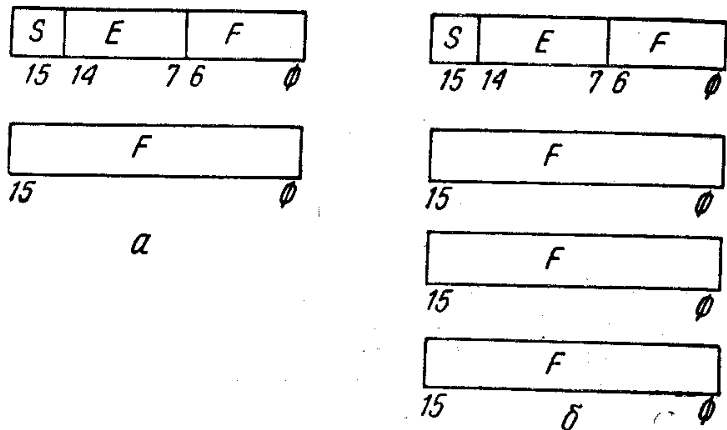
Рис. 34. Формат данных с ПЗ: а — F, обычная точность; б — D, высокая точность
