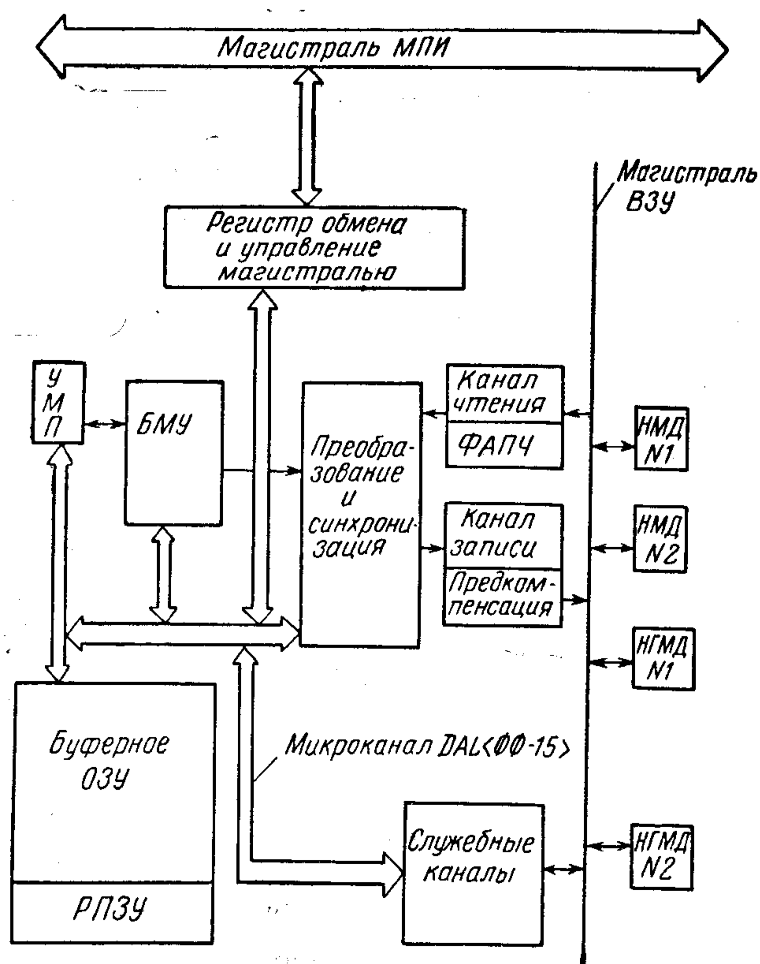
Рис. 20. Структурная схема контроллера SM 1425.5140 (ФАПЧ — схема фазовой подстройки частоты)
