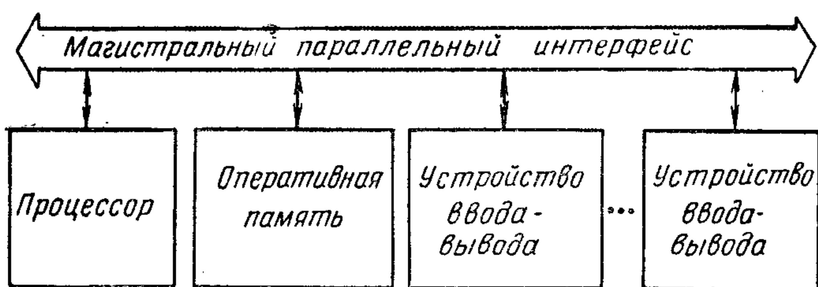
Рис. 17. Обобщенная структурная схема подключения устройств к МПИ
