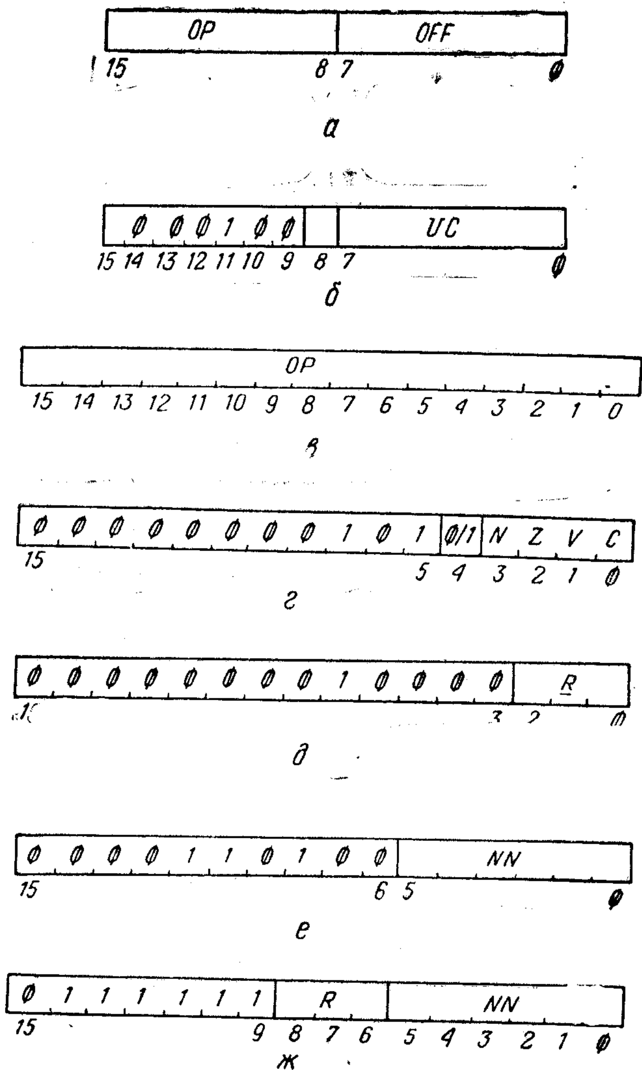
Рис. 30. Форматы команд: а — ветвлений; б — EMT, TRAP; в — безадресных RTI, BPT, IOT, RTT, MFPT; г — изменения признаков; д — RTS; е — MARK; ж — SOB
