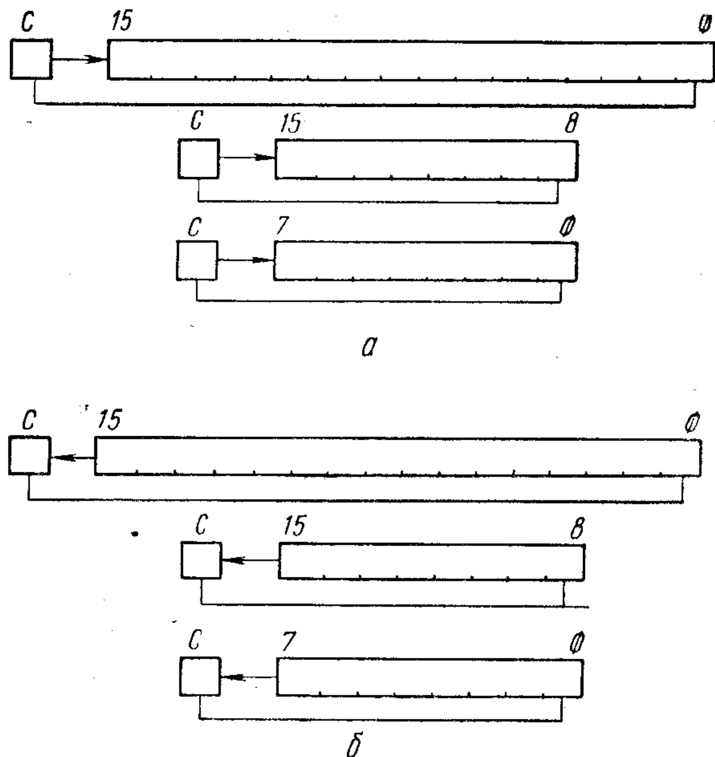
Рис. 31. Циклический сдвиг: а — вправо ROR (B); б — влево ROL (B)
