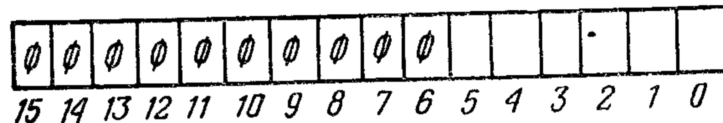
Рис. 15. Формат регистра MMR3.
