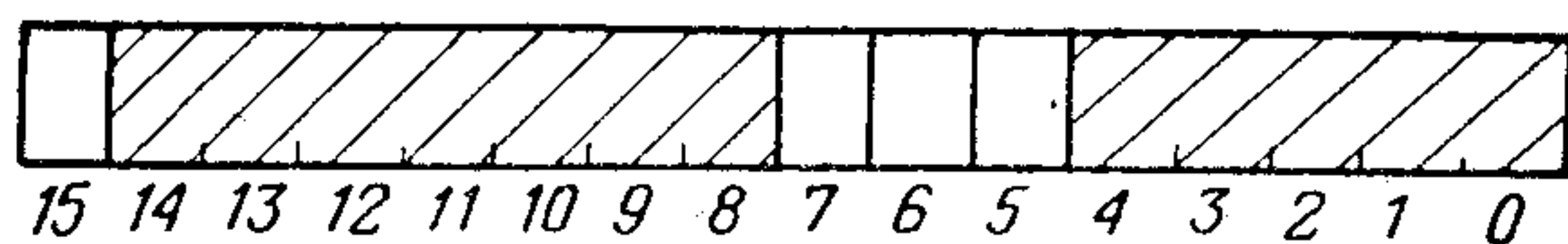
Рис. 11. Формат регистра MSER
