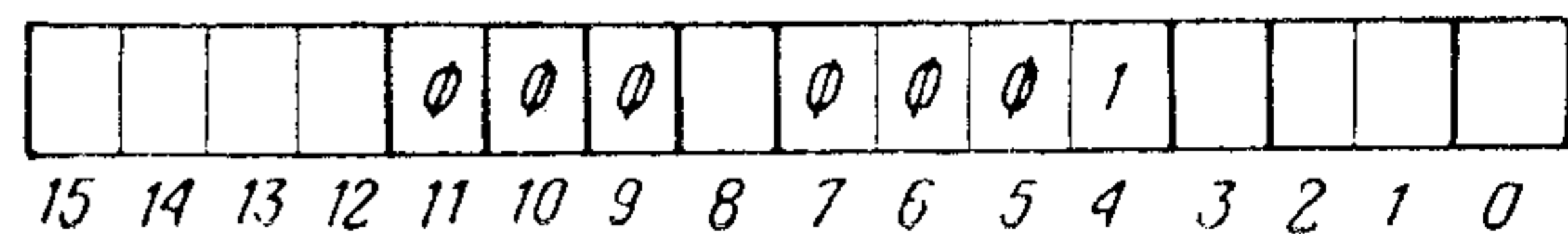
Рис. 6. Формат регистра MR
