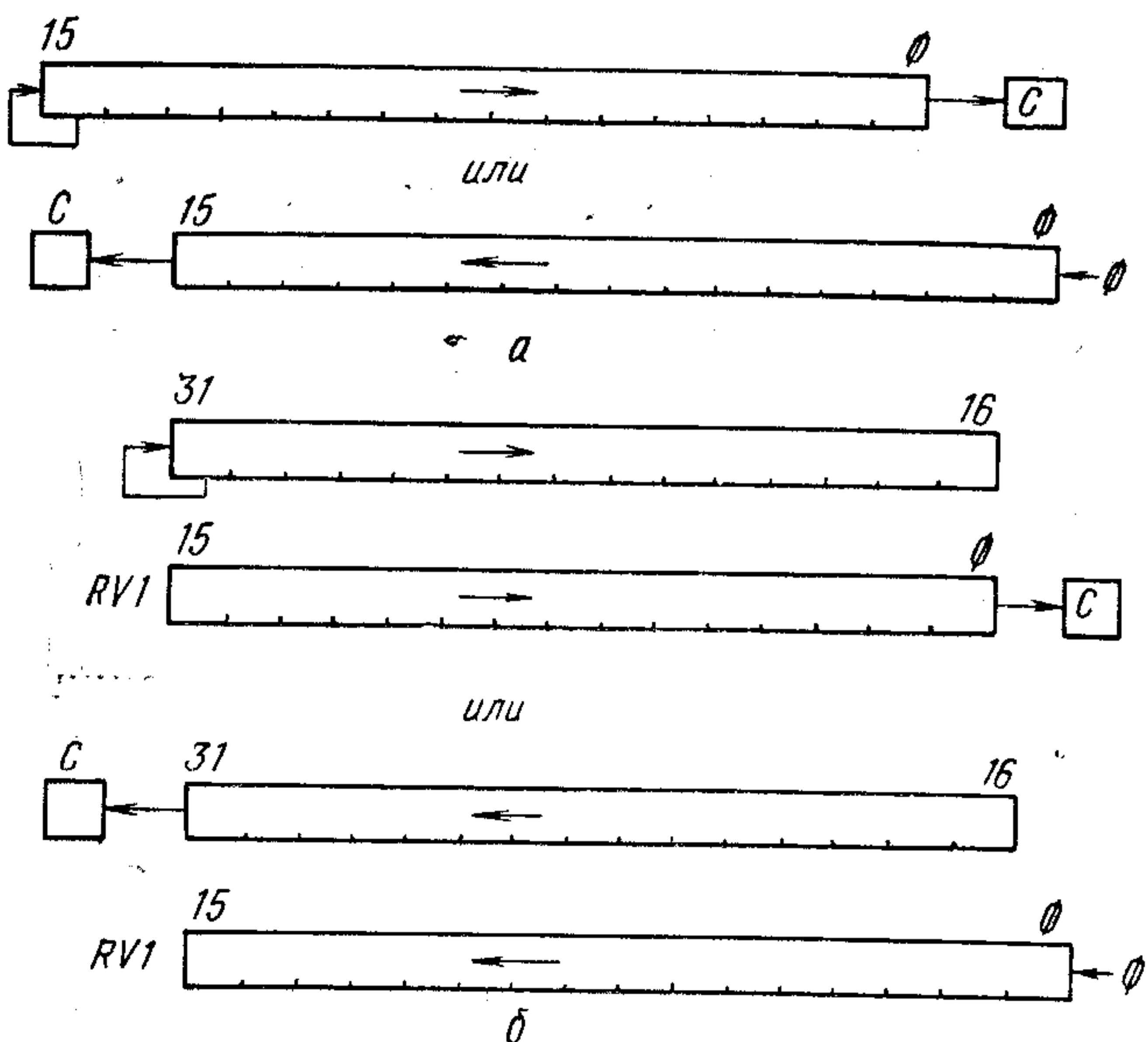
Рис. 33. Арифметический сдвиг (двухадресные команды): а — ASH; б — двойного слова ASHC
