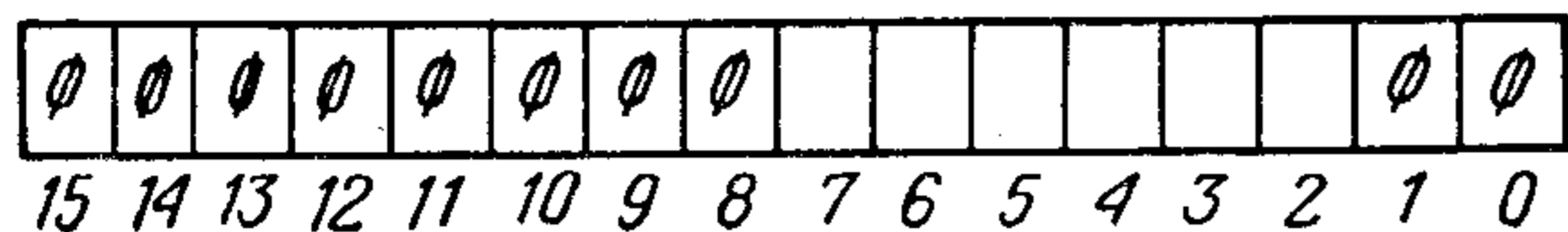
Рис. 4. Формат регистра CPUERR
