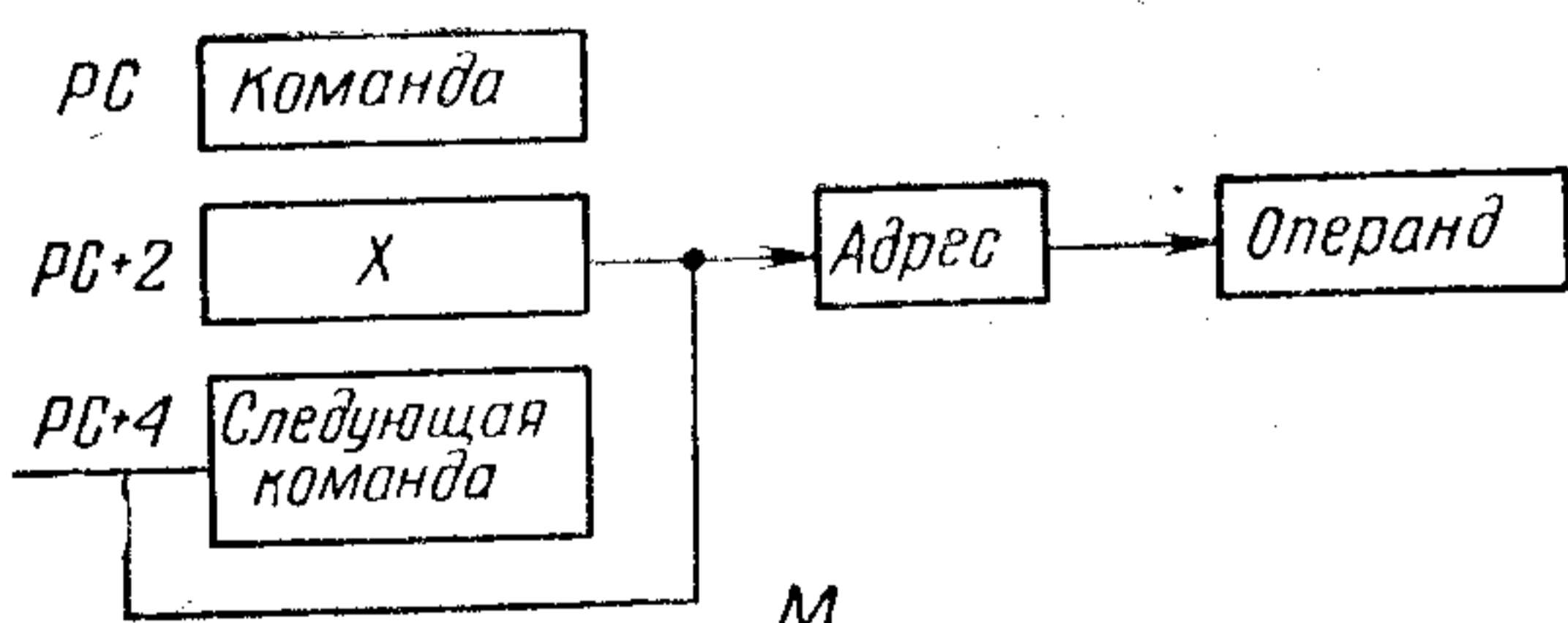
Рис. 27. Режимы адресации:
