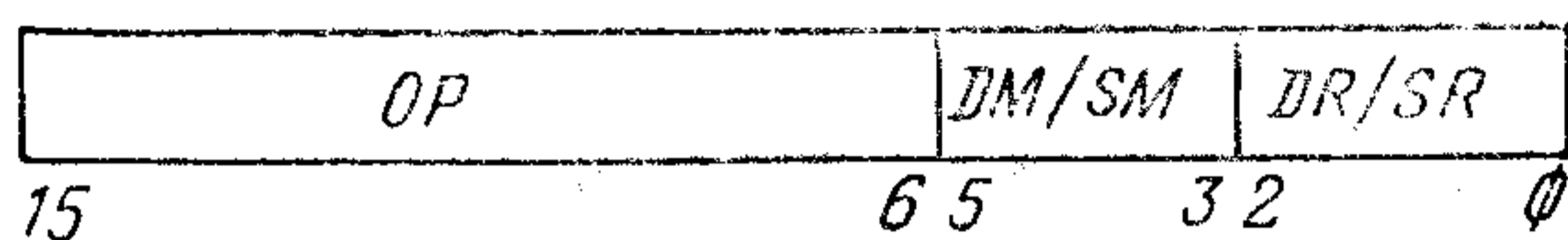
Рис. 28. Формат одноадресных команд и команды JMP
