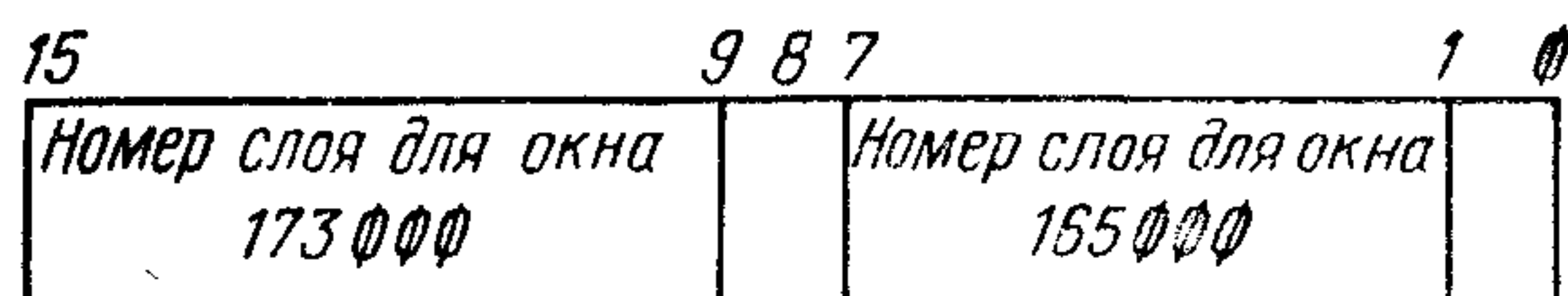
Рис. 26. Формат регистра PCR
