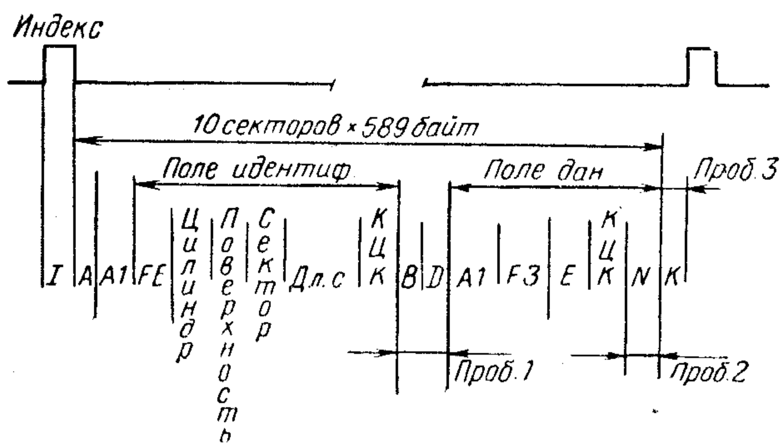
Рис. 25. Формат дорожки НГМД:
