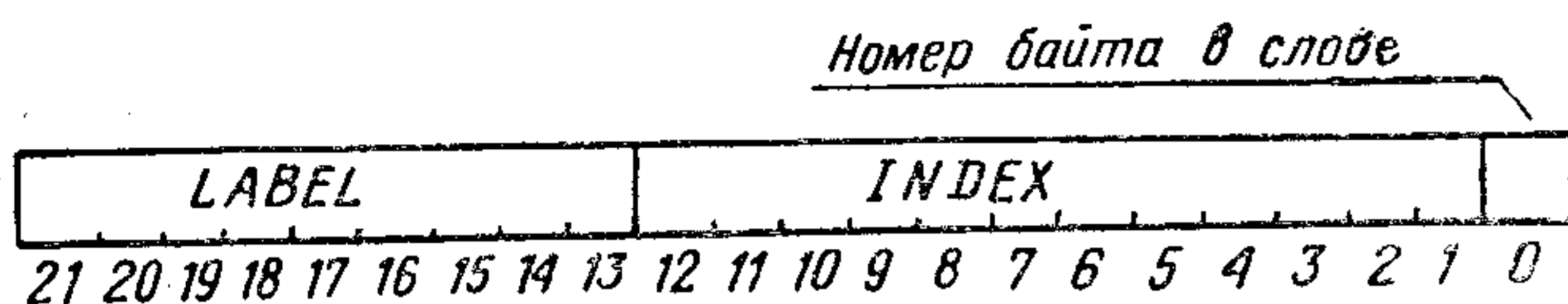
Рис. 7. Формат адреса ББП
