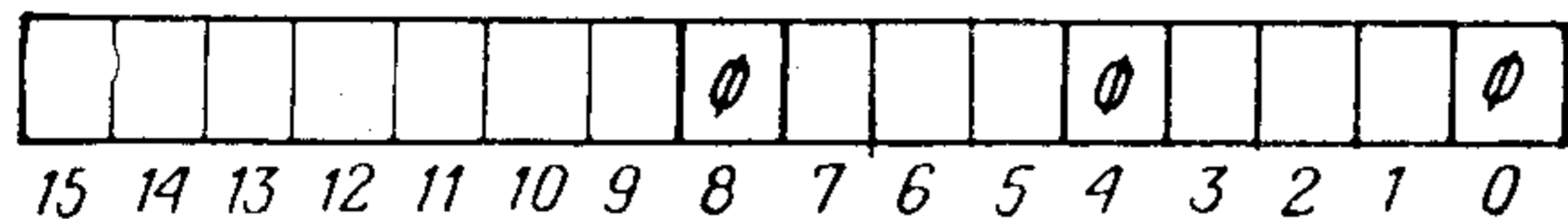
Рис. 5. Формат регистра PIRQ
