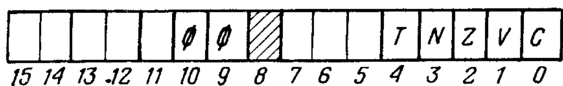
Рис. 3. Формат регистра PSW
