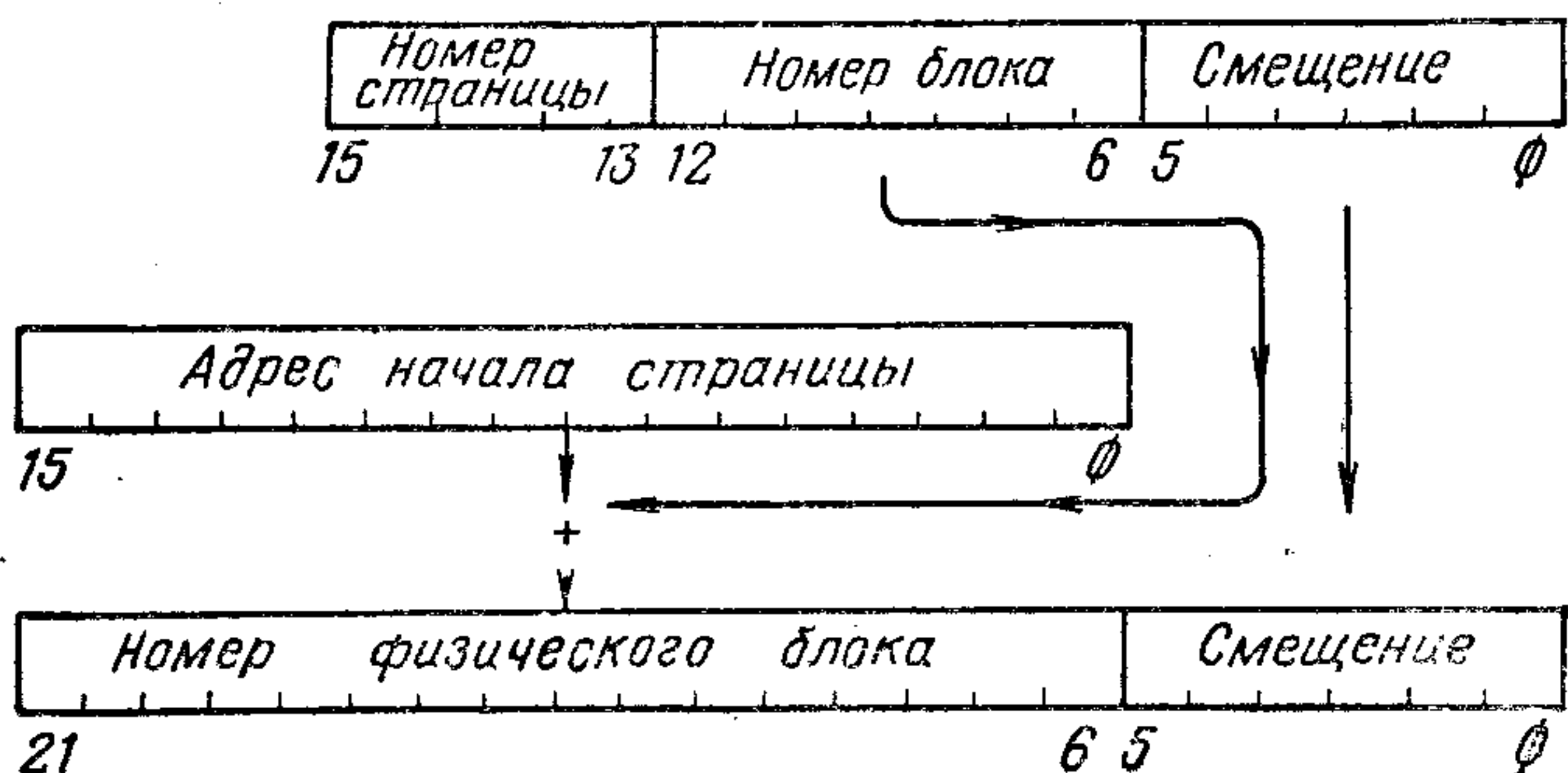
Рис. 16. Схема формирования физического адреса ДП
