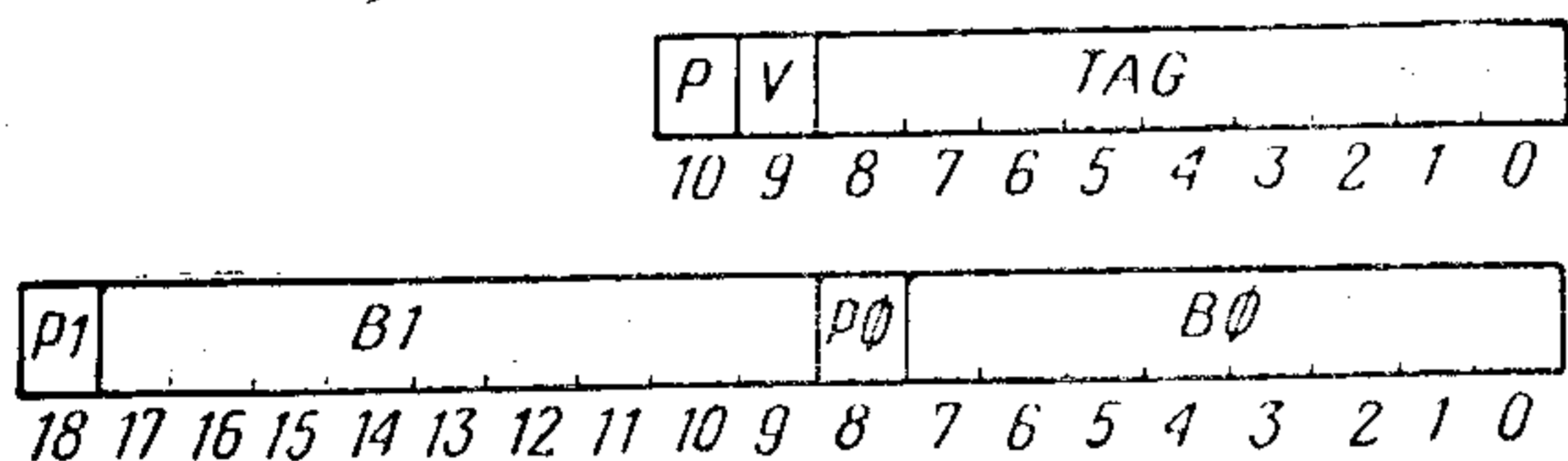
Рис. 8. Формат слова ББП
