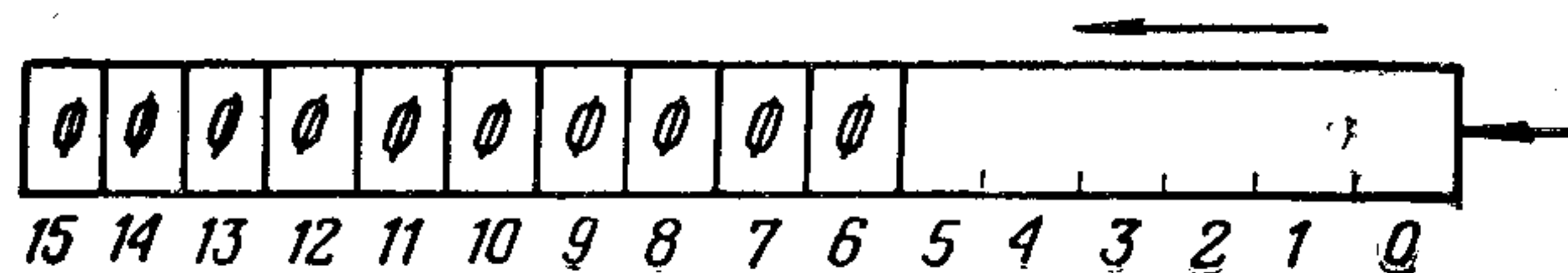
Рис. 10. Формат регистра HMR
