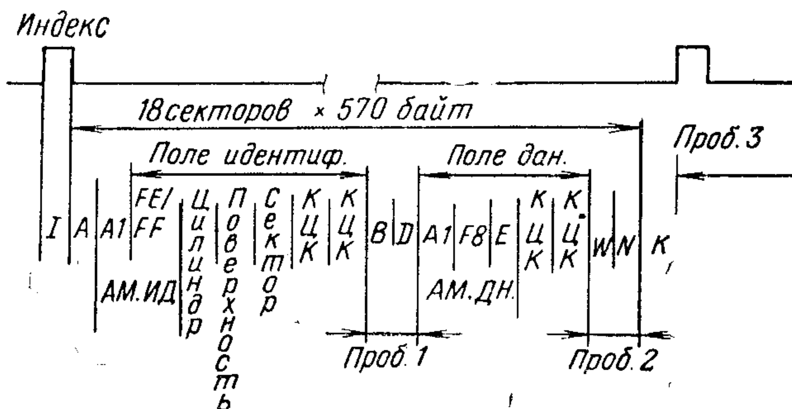
Рис. 24. Формат дорожки НМД:
