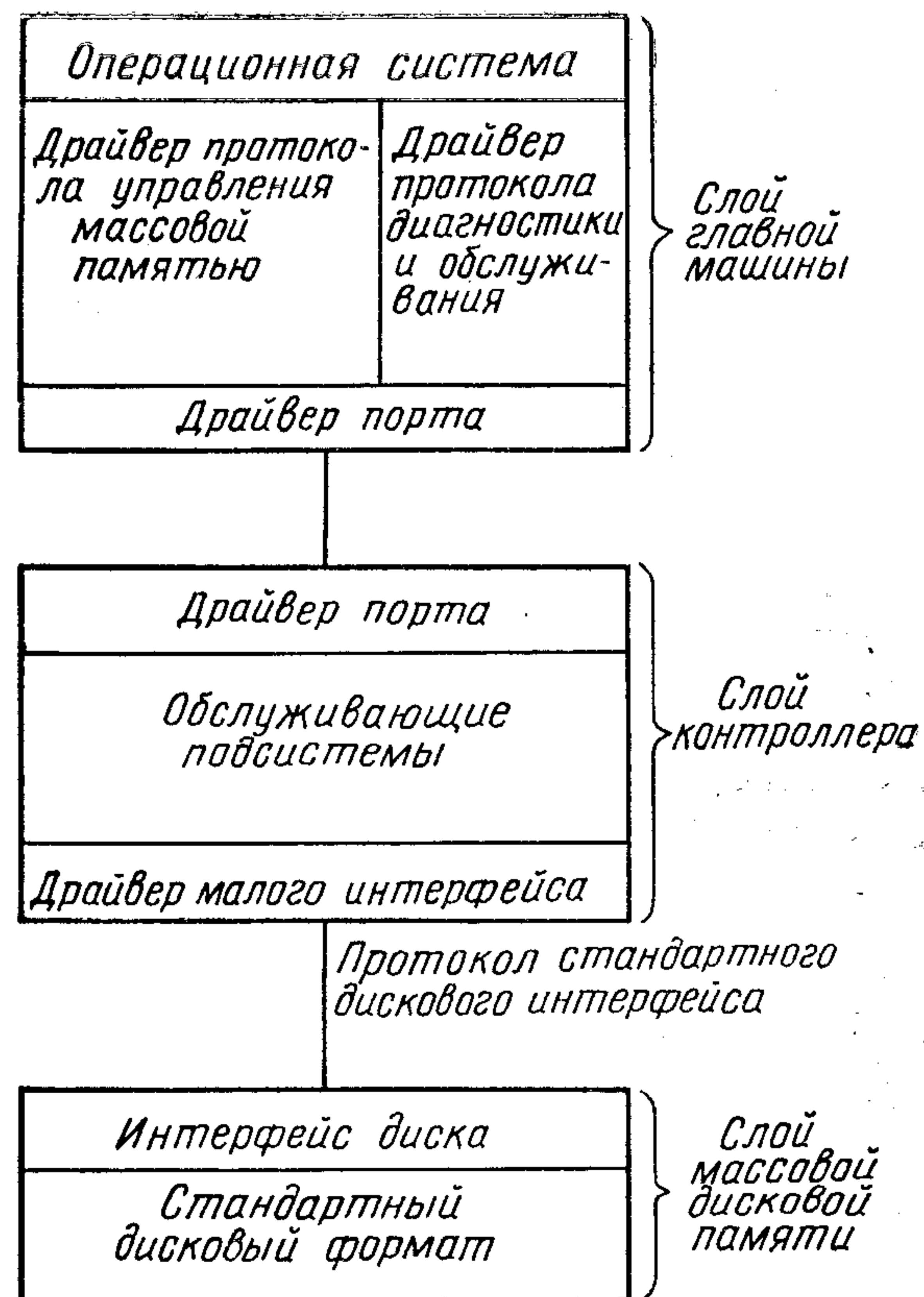
Рис. 18. Компоненты архитектуры массовой памяти слой, драйвер портов, постоянно находящийся в главном слое, передает пакеты по шине между главной машиной и контроллером.
