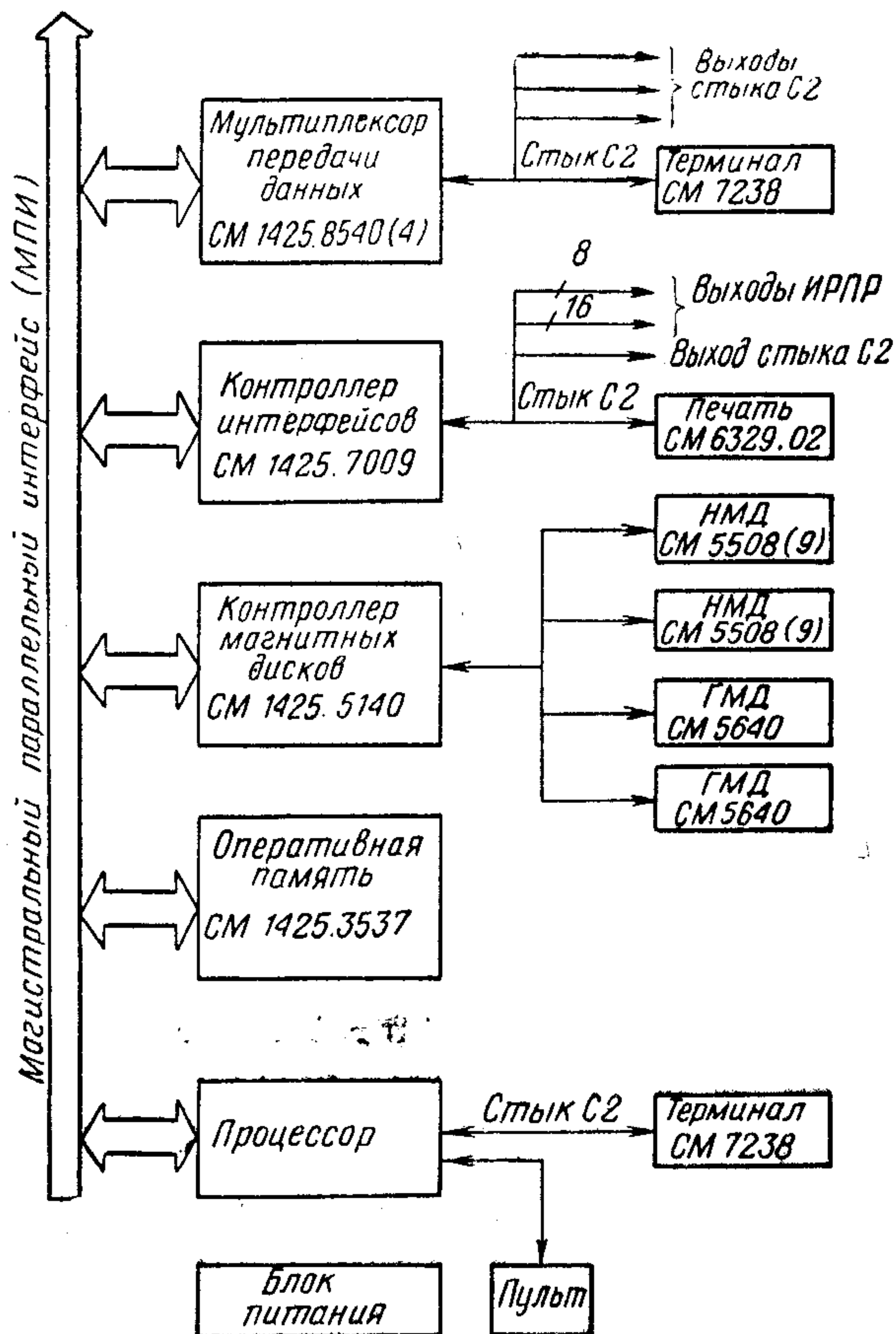
Рис. 2. Структурная схема типового комплекса СМ 1425
