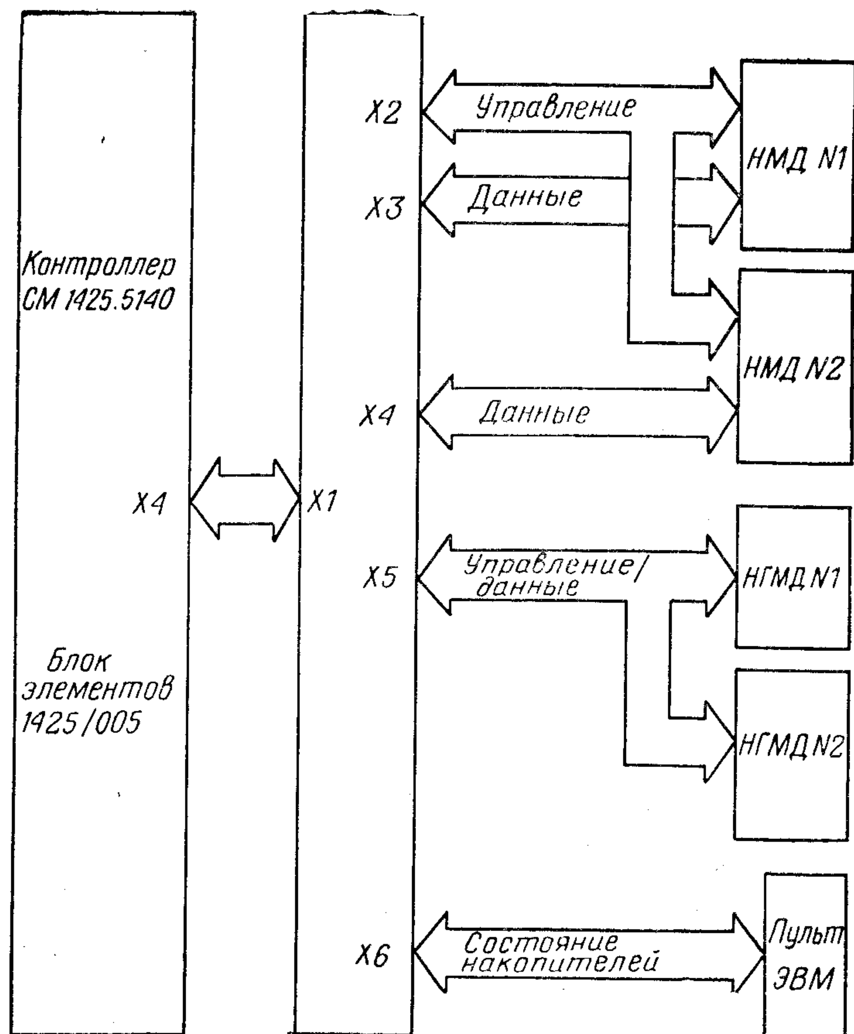
Рис. 22. Схема подключения контроллера к ВЗУ
