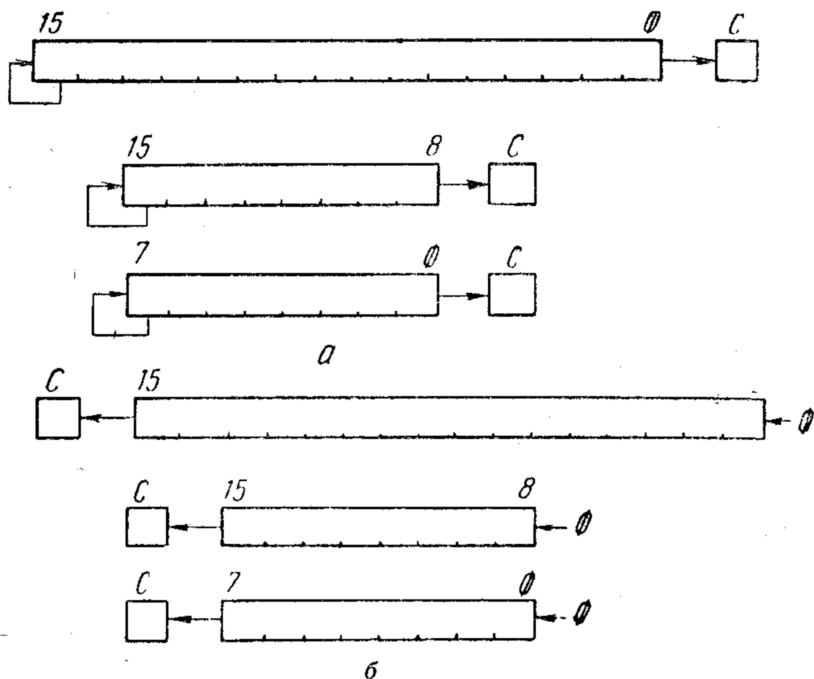
Рис. 32. Арифметический сдвиг (одноадресные команды): а — вправо ASR(B); б — влево ASL(B)
