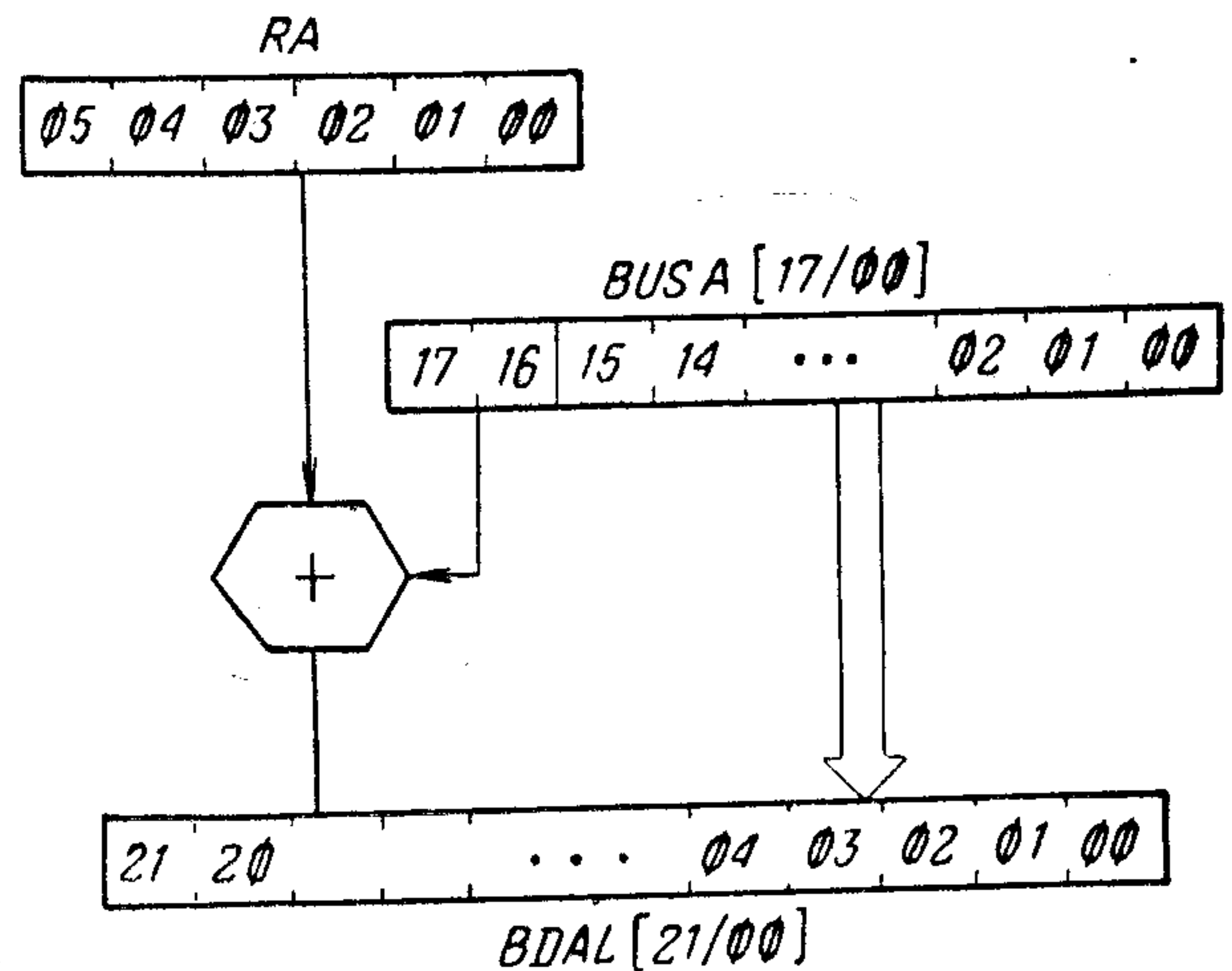
Рис. 23. Схема формирования в УССИ 22-разрядного адреса МПИ из 18-разрядного адреса ОШ
