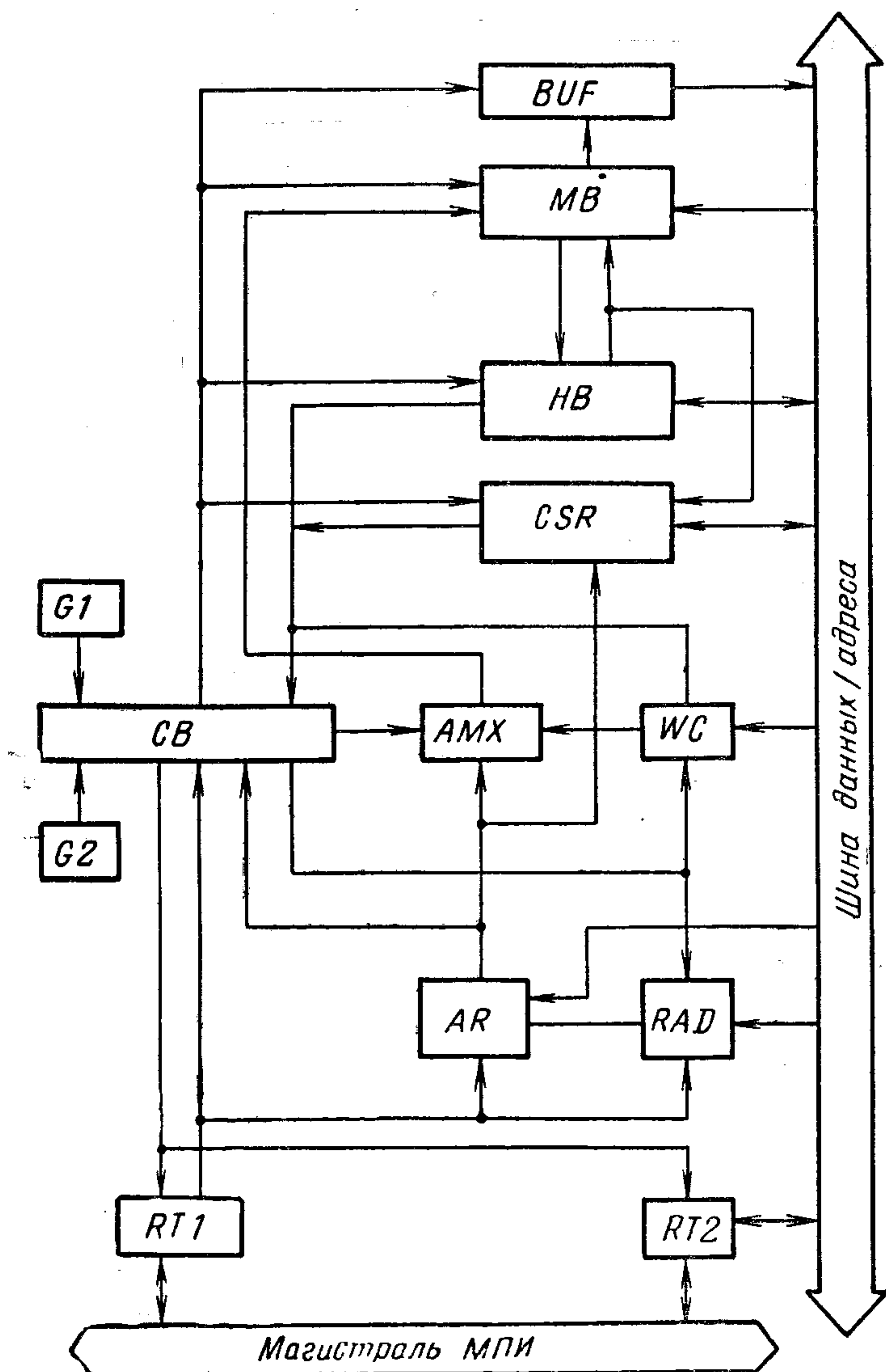
Рис. 19. Структурная схема МОЗ
