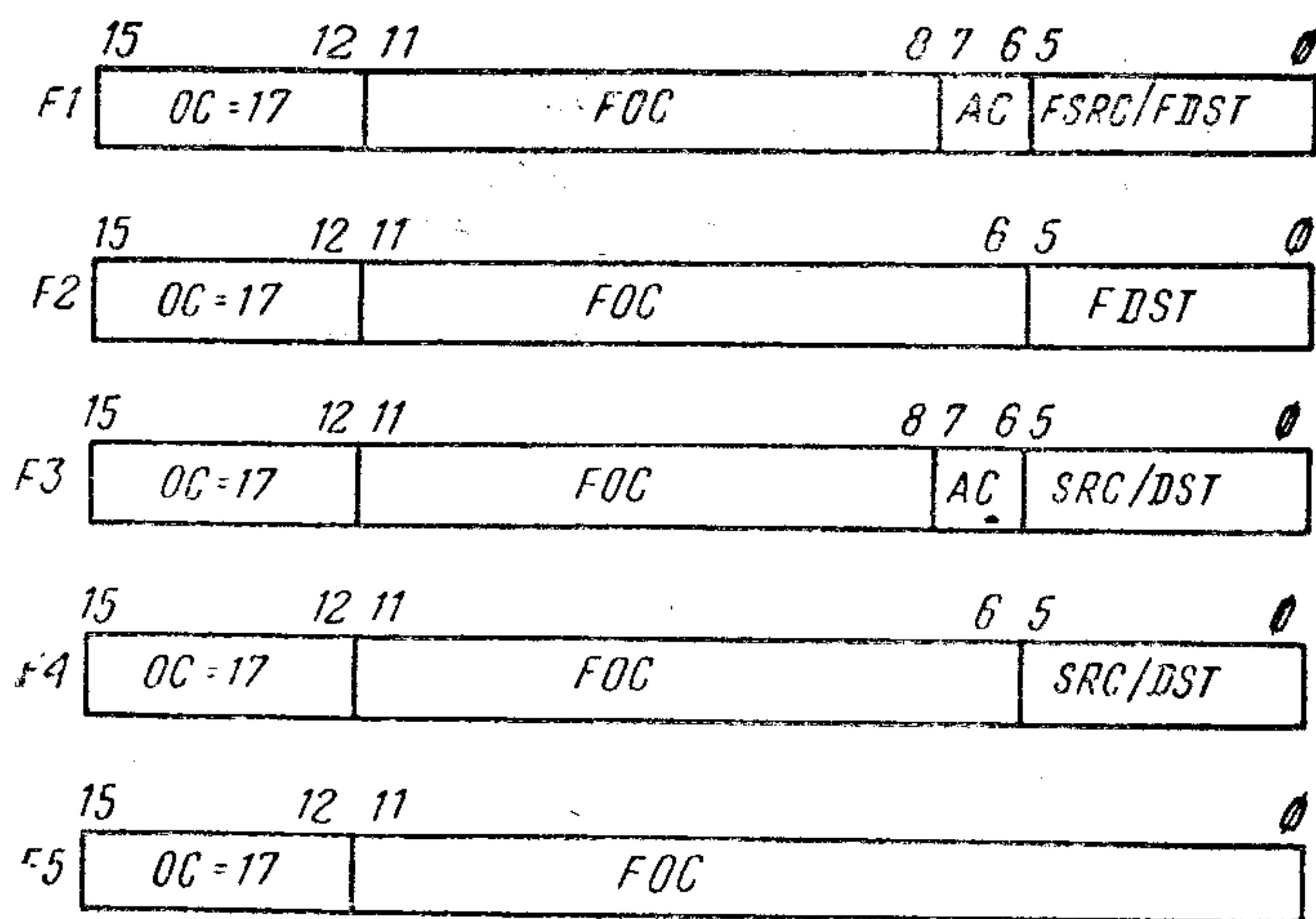
Рис. 38. Форматы команд с ПЗ
